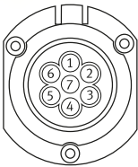
Kit Aragón 507 7 poli KAJ07B0 €. 85,00
