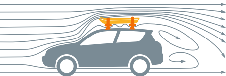
Portasci da tetto
